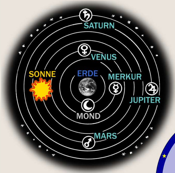
Ptolemäus
